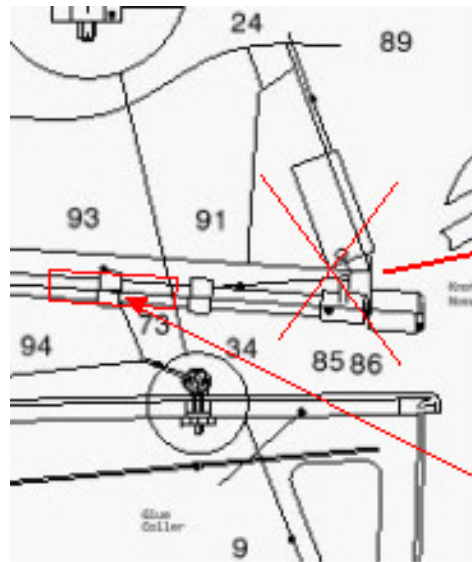
Fockbaum um 5 mm verlängern, z.B. mit einer Hülse
